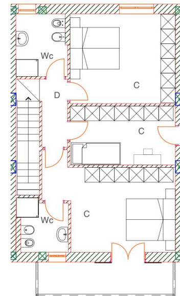
PLANIMETRIA FUORI SCALA
